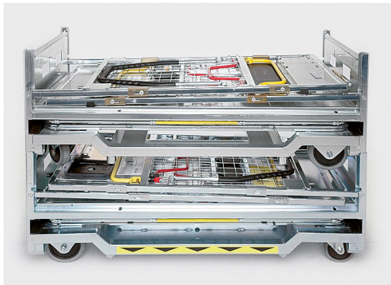
Sammelbehälter gestapelt
